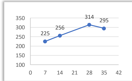
Gambar 2. Grafik kuat tekan beton 5% slag nikel
