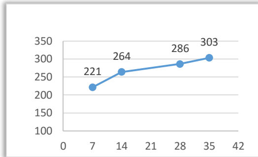
Gambar 1. Grafik kuat tekan beton normal
