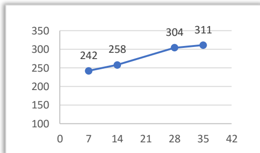
Gambar 3. Grafik kuat tekan beton 15%
